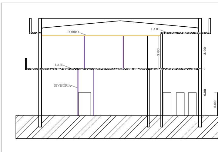
CORTE A-A ESCALA: 1:200
