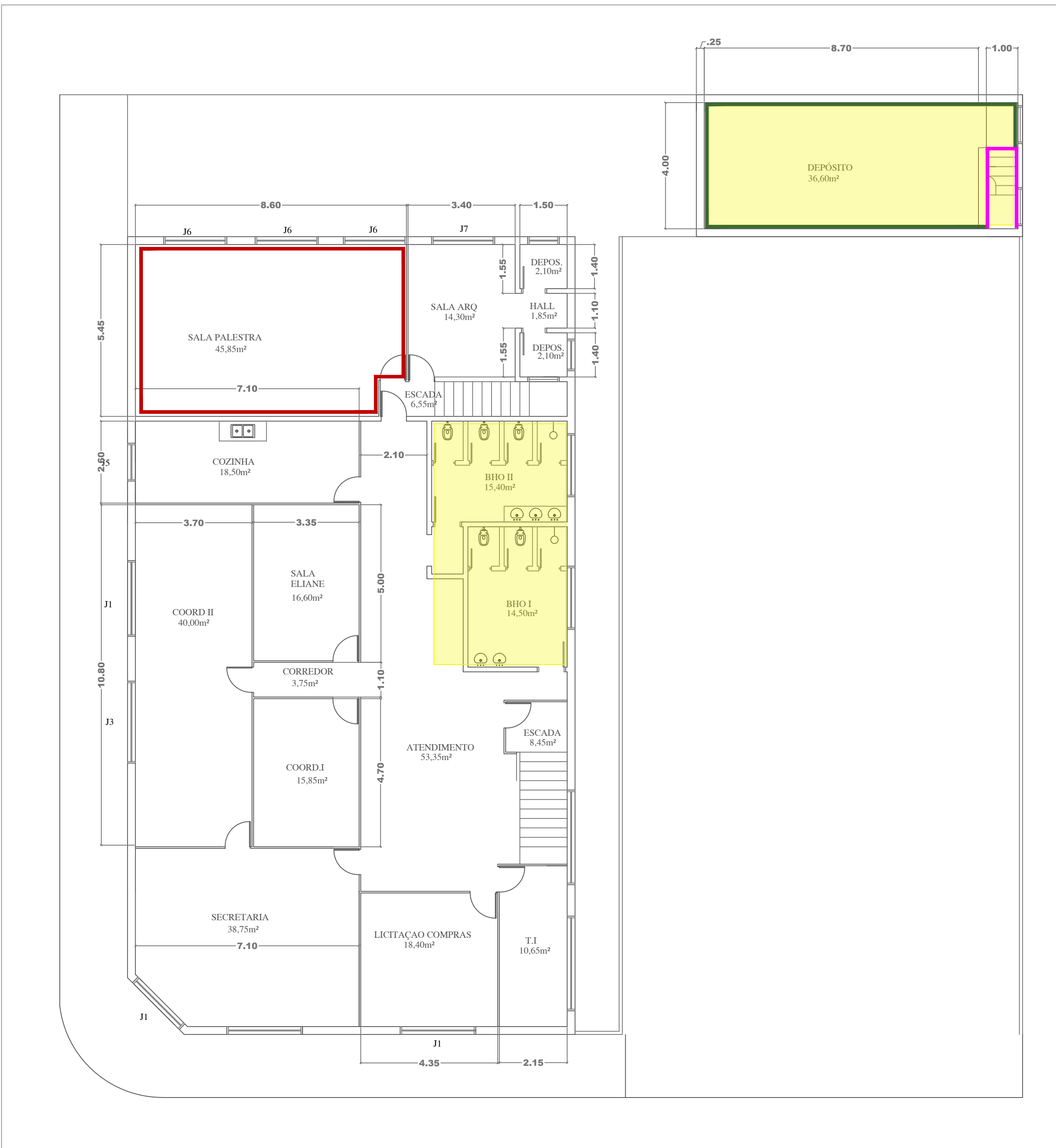
PLANTA DA EDIFICAÇÃO - PAVIMENTO SUPERIOR LOCAIS DE PINTURA ESCALA: 1:100
