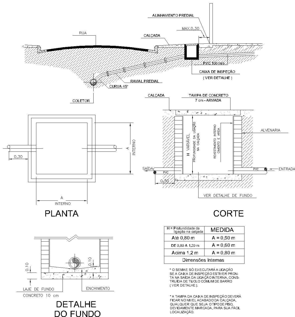
Figura 02: Detalhe da ligação de esgoto.
