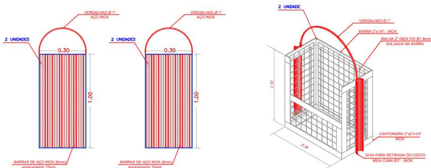
DETALHE DO CESTO E DA GRADE SEM ESCALA
